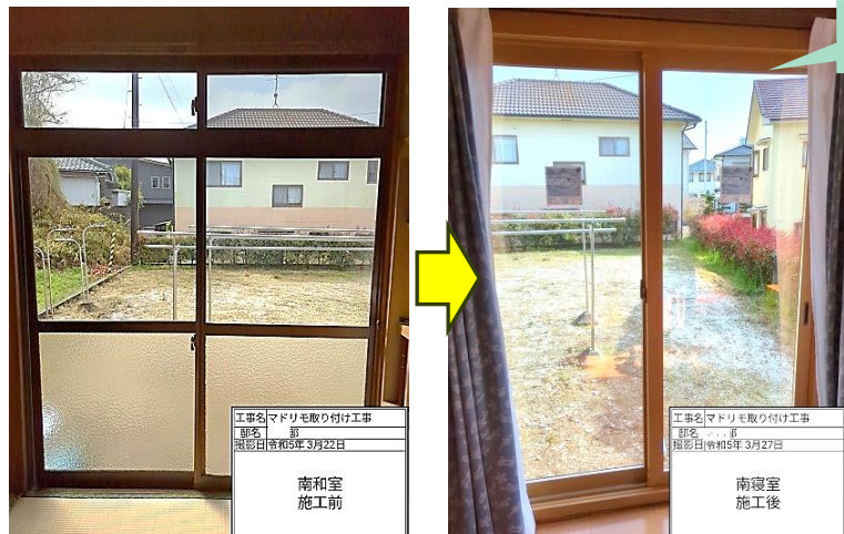
カバー工法 1,685×2,200
